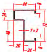
Sectie profiel
