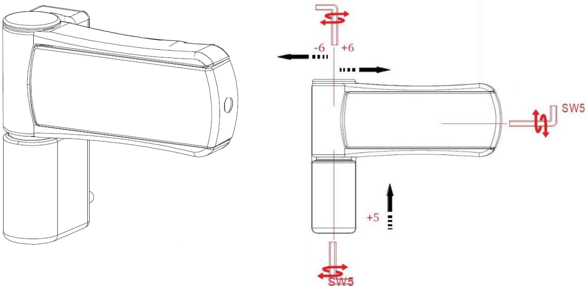
Afbeelding 3D scharnieren: af te stellen in 3 richtingen
