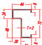
Sectie profiel
